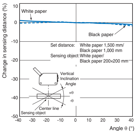
E3AS-F1500□
